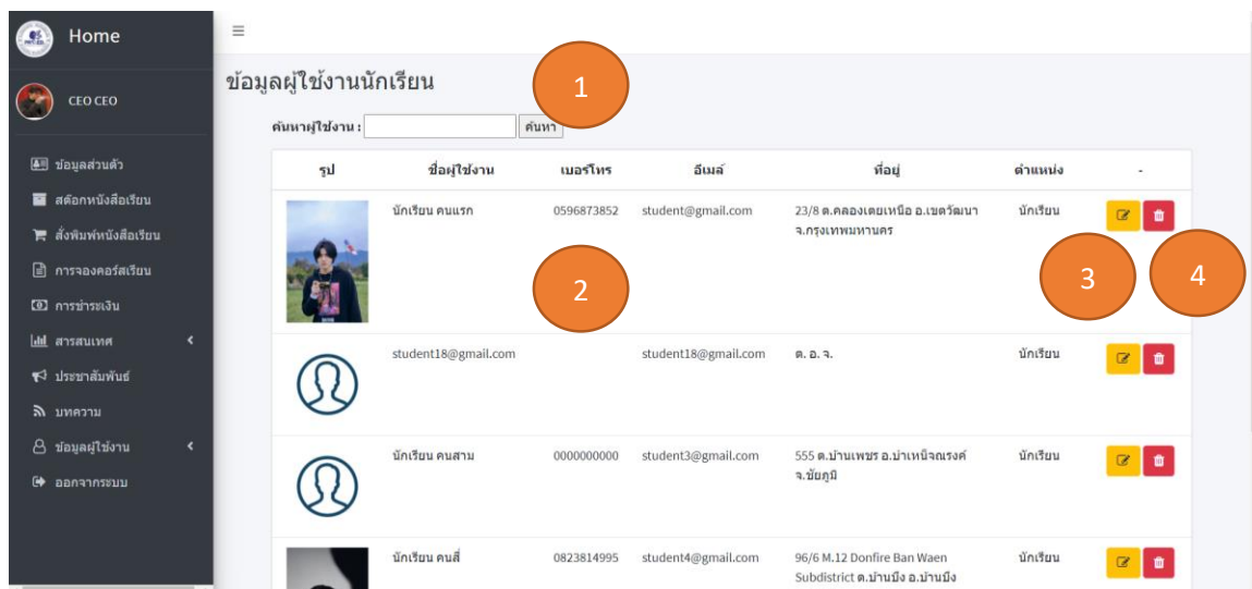
ภาพที่ ข.23 ภาพแสดงหน้าจอจัดการข้อมูลผู้ใช้งานนักเรียนสำหรับเจ้าของสถาบันกวดวิชา
